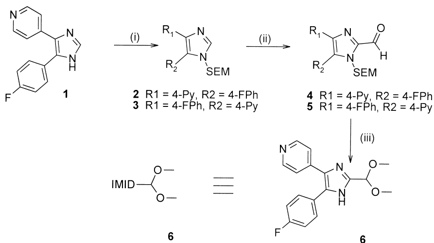
Scheme 1. Preparation of the dimethylacetal 6 . (i) (CH 3 ) 3 SiCH 2 CH 2 OCH 2 Cl, NaH, DMF; (ii) BuLi, N -formylmorpholine, THF; (iii) methanol, HC(OCH 3 ) 3 , p -toluenesulphonic acid.
